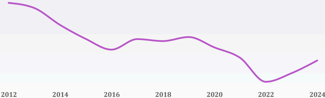
Flare trend
